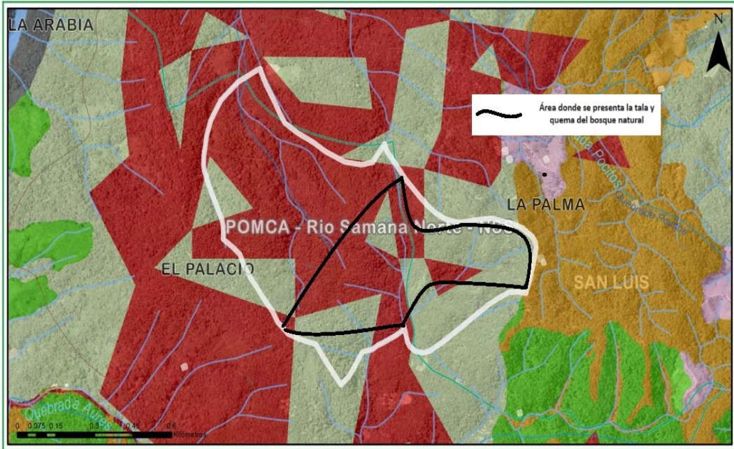
Figura 3. Zonificación ambiental del predio con PK 6602001000003400056 Fuente: Geoportal corporativo, 2024
