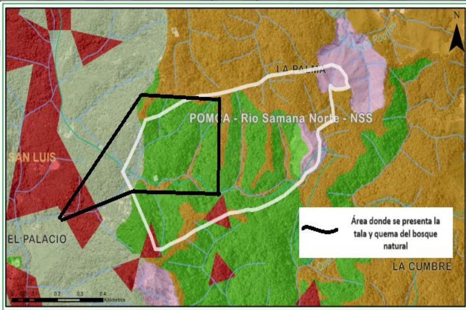
Figura 4. Zonificación ambiental del predio con PK 6602002000001200003. Fuente: Geoportal corporativo, 2024
