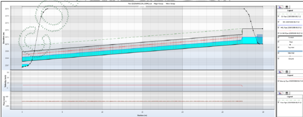
FIGURA 28-Gráfico de evolución del caudal en el modelo hidráulico, t=27:12 (Estable)
