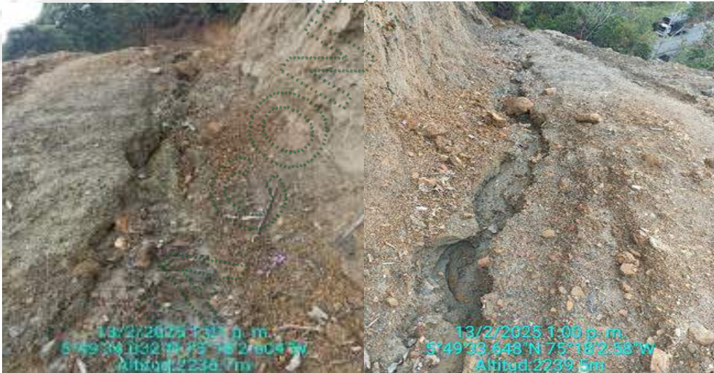
Grietas en la base del talud de corte
