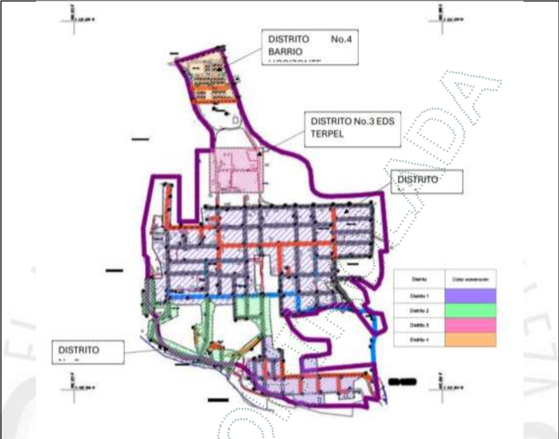
Imagen 1. Sistema de alcantarillado existente Corregimiento de Puerto Perales, Municipio de Puerto Triunfo
