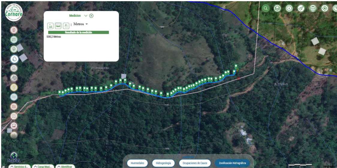
Figura 1. Tramo por donde se había aperturado una vía que comunica las veredas La Gaviota, Los Planes, Santa Rita del municipio de San Luis Tomado del Geoportal Interno MapGis Cornare 2024
