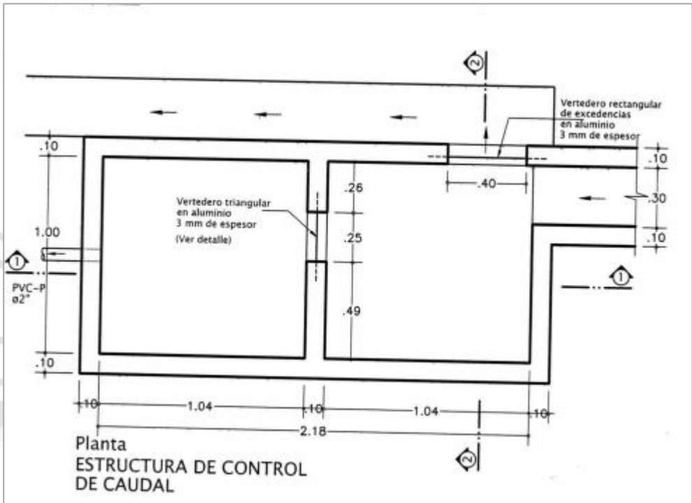
Imagen 1. Diseño obra de control
