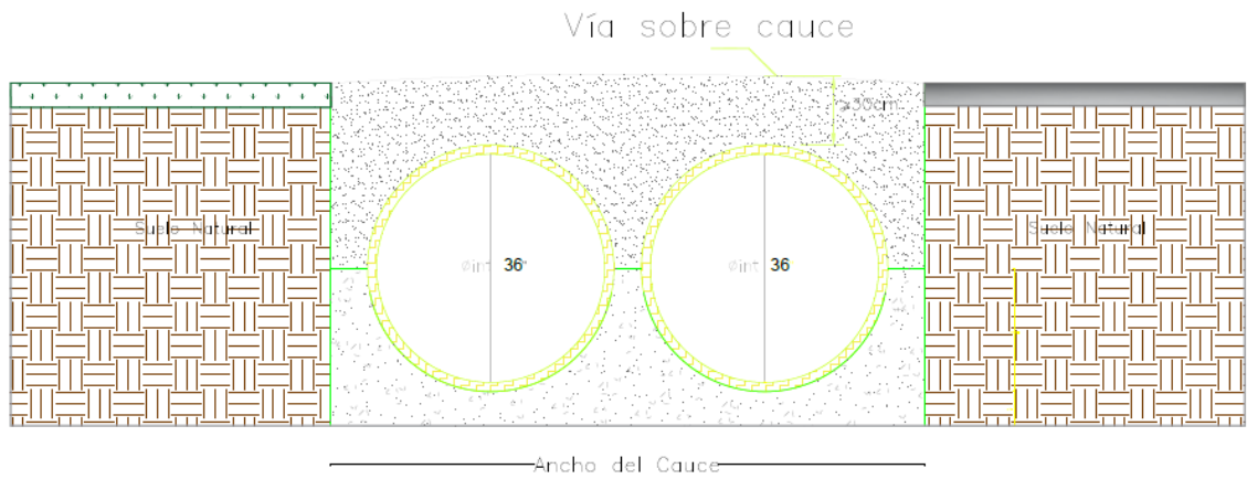
INSTALACIÓN DE DUCTO ESQUEMA GENERAL
