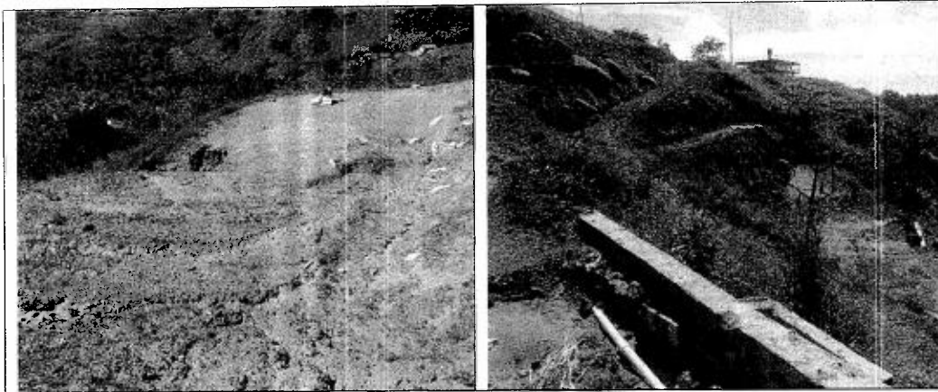
Imágenes 19 y 20. Corte de taludes con alturas superiores a 3 metros de altura, que por falta de obras drenaje arrastra sedimentos a las fuentes cercanas.
