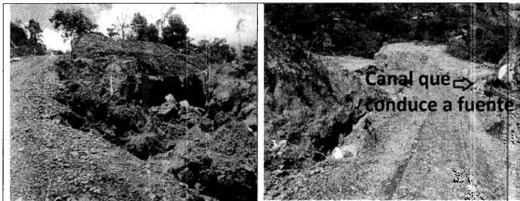
Imágenes 21 y 22. Proceso erosivo tipo cárcavas y corte de taludes, que afecta una corriente.
