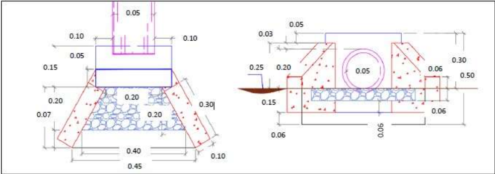
Imagen No: diseño de obra de descarga
