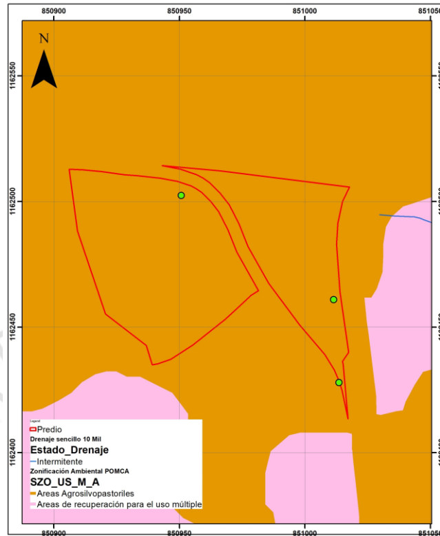
Imagen 1: Zonificación ambiental del predio según el POMCA.
