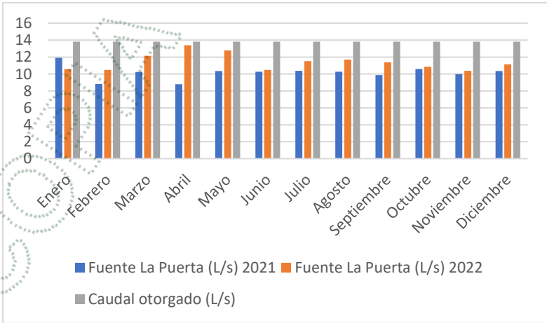
Figura 2. Consumos del año 2021 y 2022 y caudal otorgado de la fuente La Puerta
