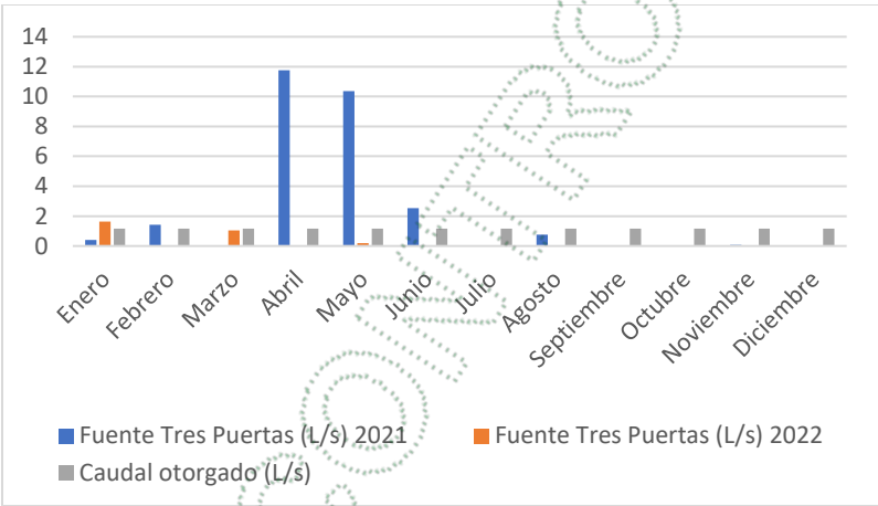
Figura 1. Consumos del año 2021 y 2022 y caudal otorgado de la fuente Tres Puertas
