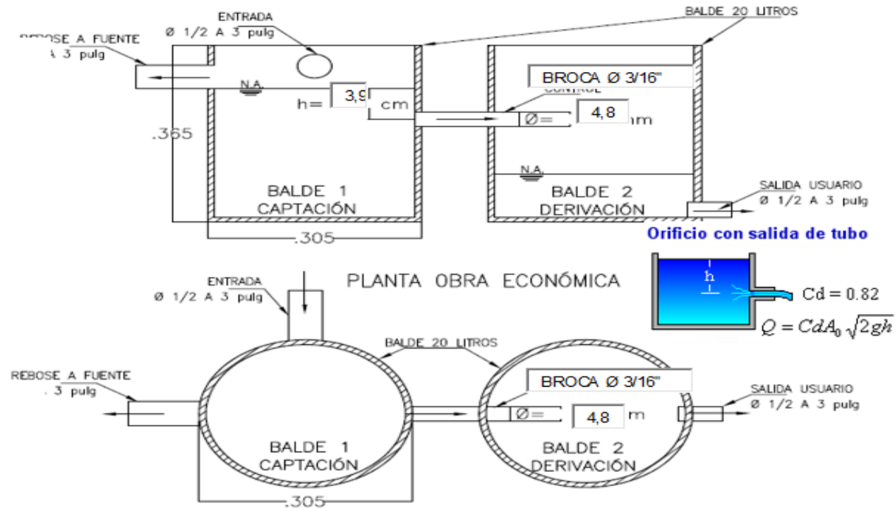
CORTE OBRA ECONÓMICA
