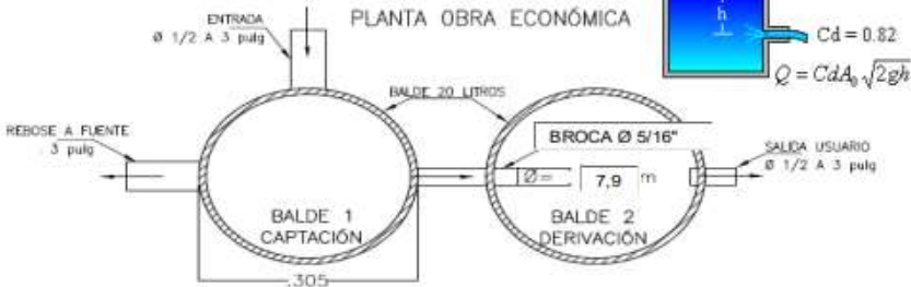
PLANTA OBRA ECONÓMICA
