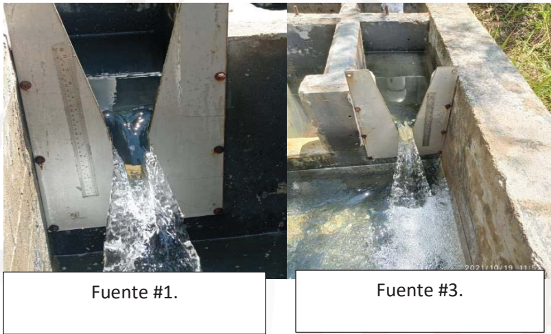
Figura 2. Vertederos triangulares para la regulación del caudal a captar.
