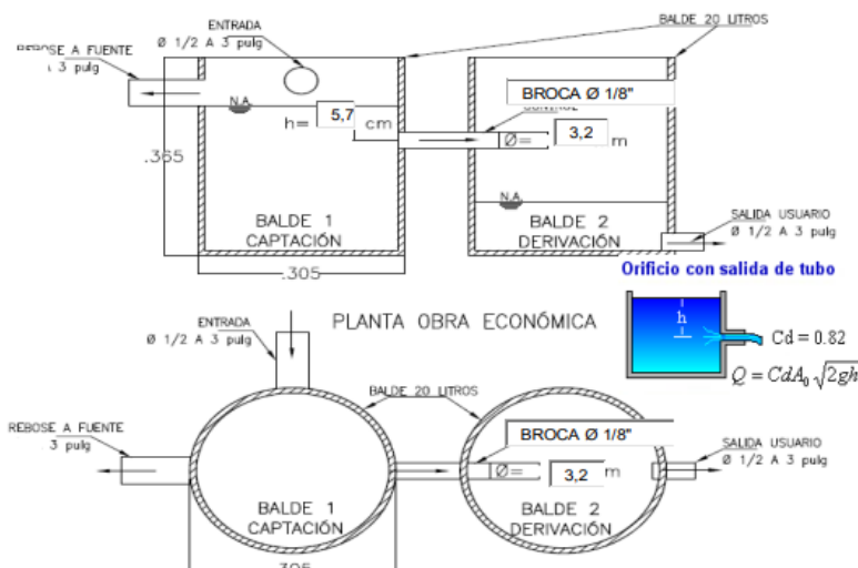
CORTE OBRA ECONÓMICA
