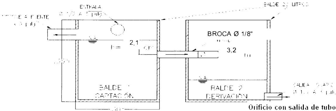
CORTE OBRA ECONÓMICA
