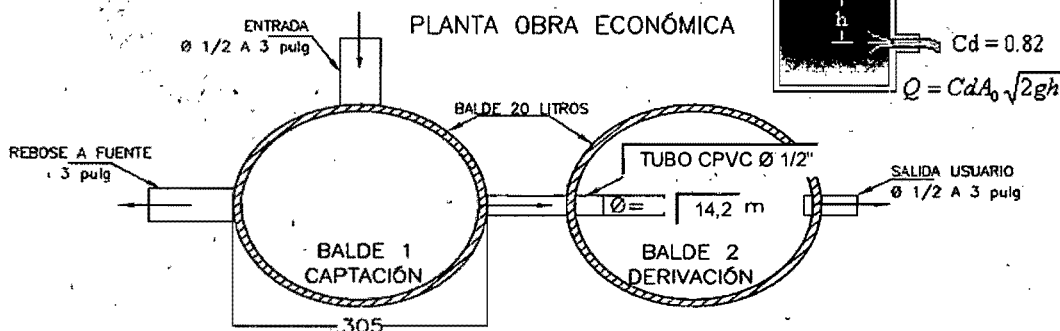
Orificio con salida de tubo
