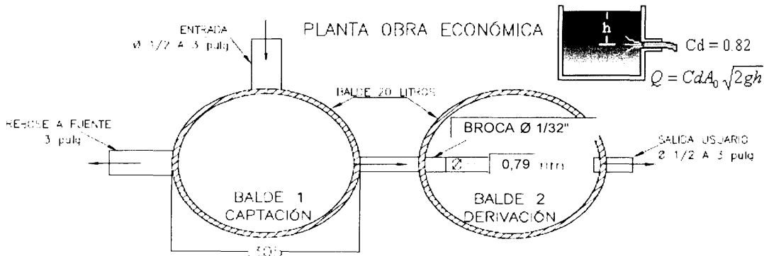
Orificio con salida de tubo
