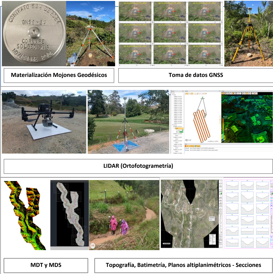
Figura 4. Actividades de la Topobatemetría realizada en las quebradas La Palma – El Salado
