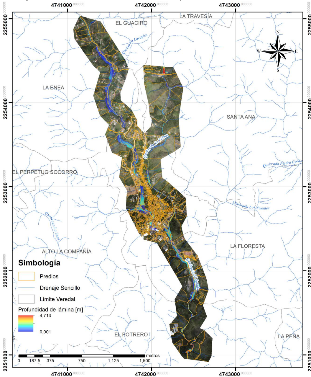
Figura 42. Mancha de inundación asociada a período de retorno de 2.33 años
